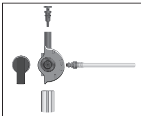
Profi-Cappuccino-Düse
